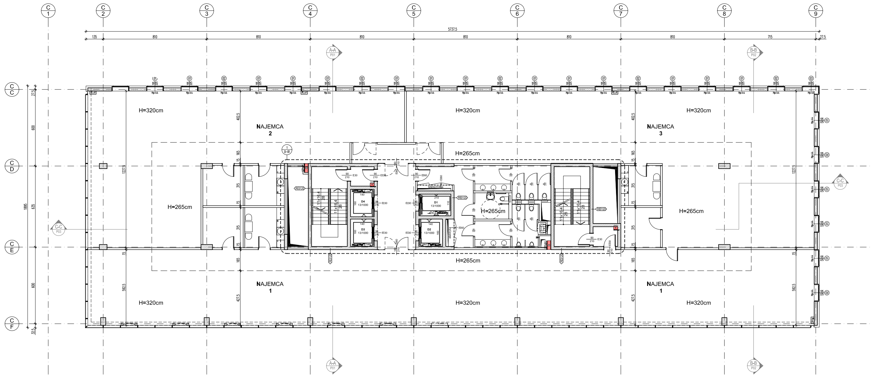
RZUT PIĘTRA TYPOWEGO (1-7) 3 najemców
